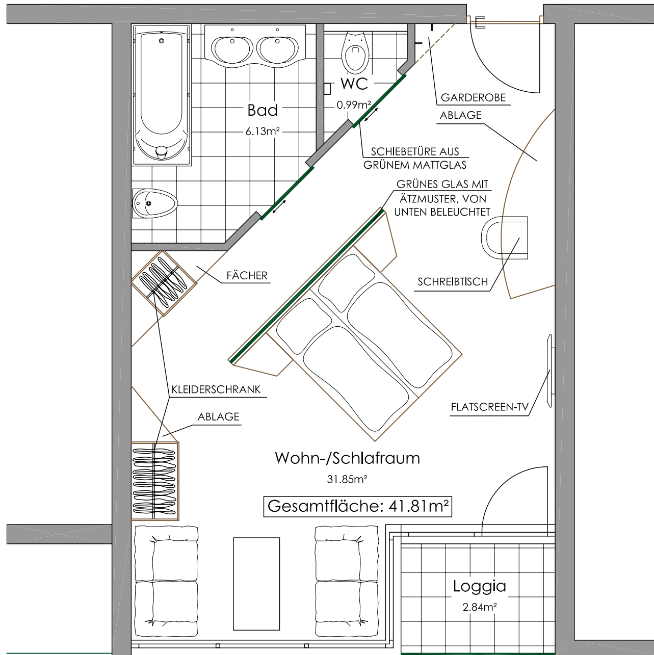
GRUNRISS 1:50
